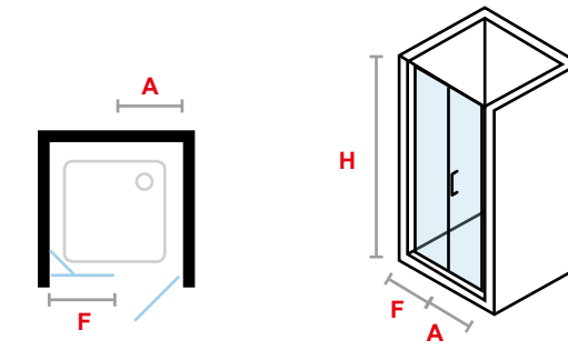
05 Puerta abatible + fijo en línea. Folding door + linear panel. Klapptür + Frontpaneel. Porte pliante + panneau linéaire. Porte pieghevoli + pannello lineare.
