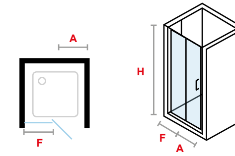
06 Puerta abatible + fijo. Panel + folding door. Panneau + Klapptür. Pannello + porte pieghevoli.
