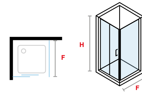
04 Puerta corredera más fijo más lateral fijo. More fixed more fixed lateral sliding door. Schiebetür + Frontpaneel + Seitenpaneel. Porte coulissante, panneau fixe et côté fixe. Porta scorrevole, porta fissa e porta laterale fissa.
