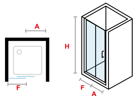
02 Puerta corredera más fijo en frontal. Sliding door plus fixed front panel. Schiebetür + Frontpaneel. Porte coulissante et panneau frontal fixe. Porta scorrevole + porta frontale fissa.
