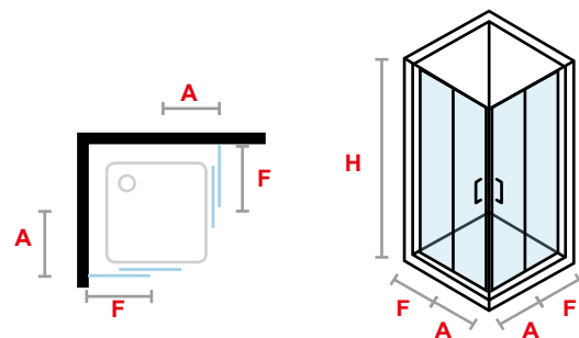
01 2 puertas correderas más 2 fijos en vertice. 2 sliding doors + 2 fixed corner panels. 2 Schiebetüren + 2 Vertex-Paneele. 2 portes coulissantes + 2 panneaux fixes en vertice. 2 porte scorrevoli + 2 porte fisse al vertice.
